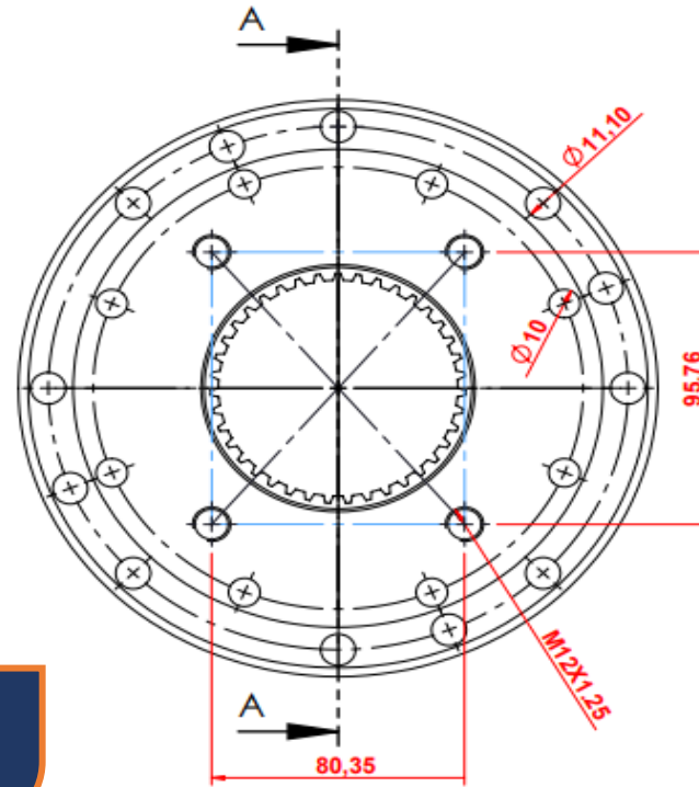
1.12.58 \Phi 203 Z39 133 246 ÇOK DELİKLİ KAPLİN/PERFORATED COUPLING
