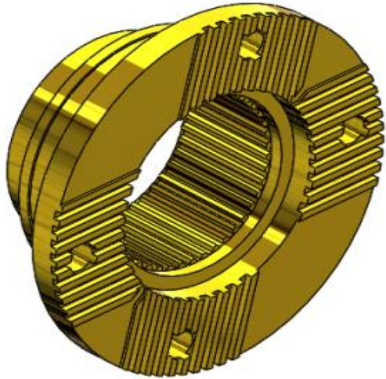
1.12.64 Q180 Z44 265 TARAMALI KAPLİN COUPLING
