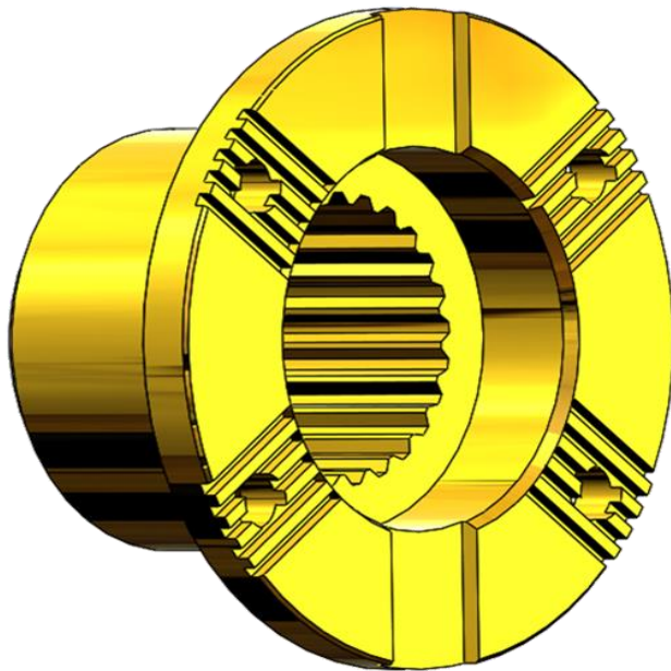
1.12.40 \Phi 180 Z:25 214 259 KAPLIN/CAPLING
