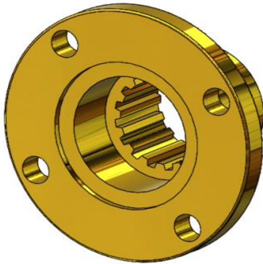
1.12.69 Ø120 Z.16 184 4 DELİK KAPLİN/COUPLING
