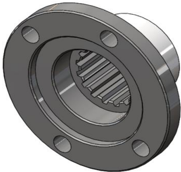
1.12.70 \Phi 120 Z.16 178-184-238-284 Kaplin/COUPLING
