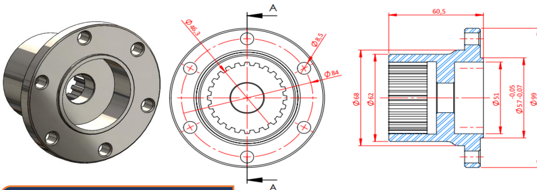
1.12.65 Ø100 Z:24 6 Delik Kaplin/COUPLING
