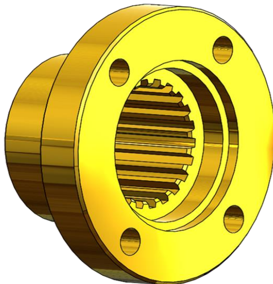
1.12.38 \varnothing 100 Z:22 KAPLIN/CAPLING
