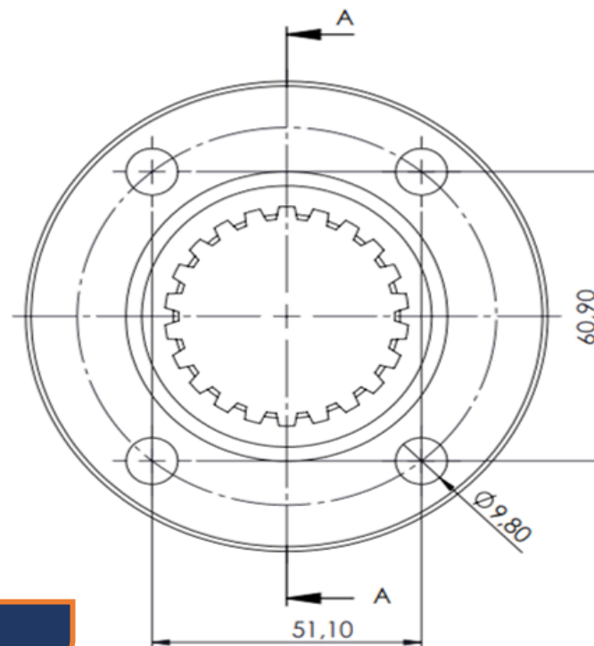
1.12.38 \varnothing 100 Z:22 KAPLIN/CAPLING
