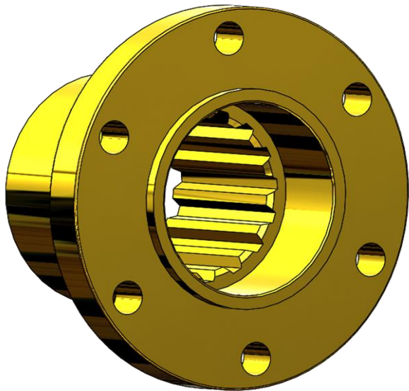
1.12.50 \varnothing 100 Z:16 244 KAPLİN/CAPLING
