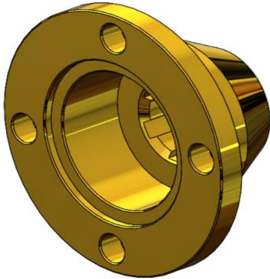
1.12.61 \phi 100 6x26x30 4 DELİK 019 UZUN KAPLIN/COUPLING
