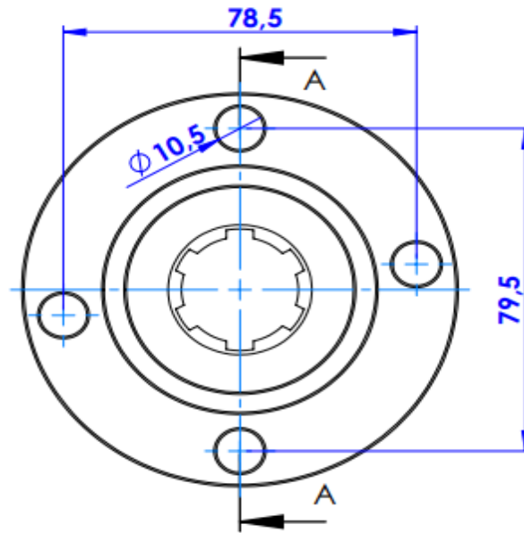
1.12.61 \phi 100 6x26x30 4 DELİK 019 UZUN KAPLIN/COUPLING
