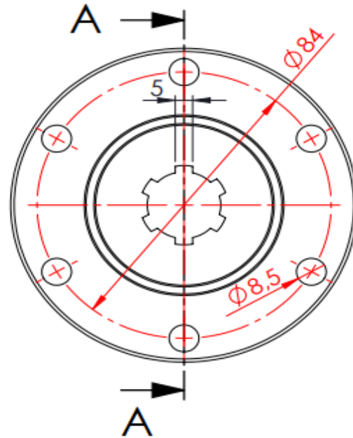
1.12.60 \phi 100 6x21x25 6 DELİK 019 UZUN KAPLİN/COUPLING
