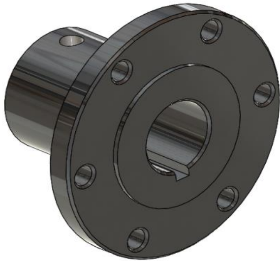
1.12.55 Ø100 6 delik Su pompası kaplini WATER PUMP COUPLING
